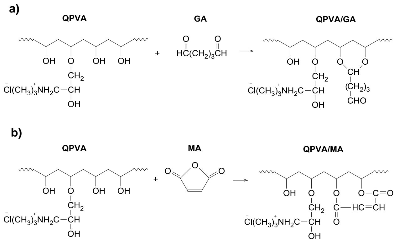
Figura 40 – Representação esquemática das reações a) QPVA e glutaraldeído e b) QPVA e anidrido maleico.
