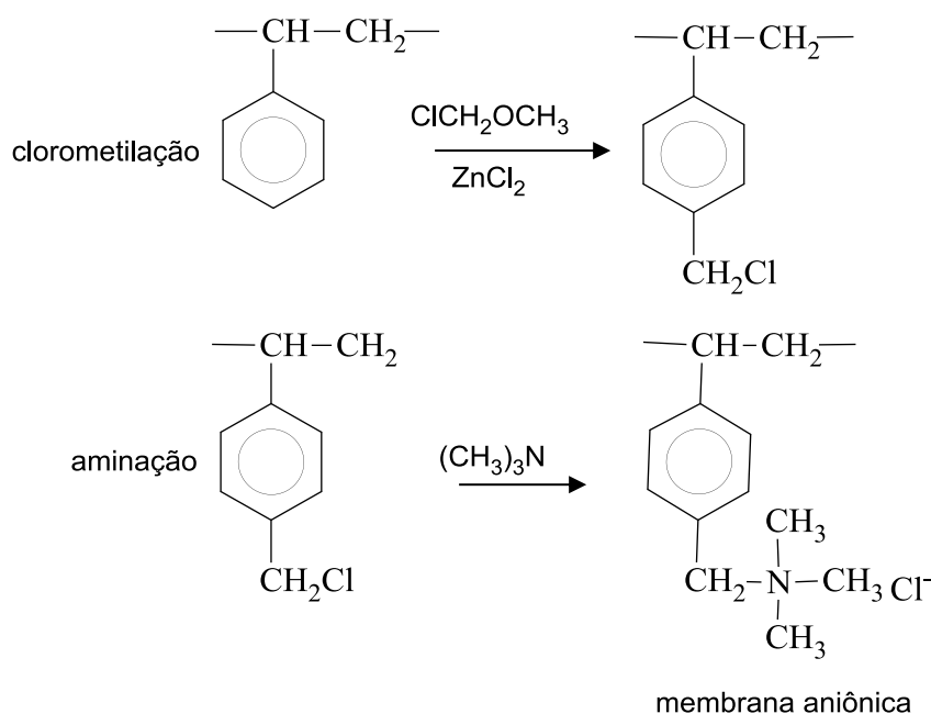
Figura 5 – Etapas para obtenção de uma membrana aniônica [40].
