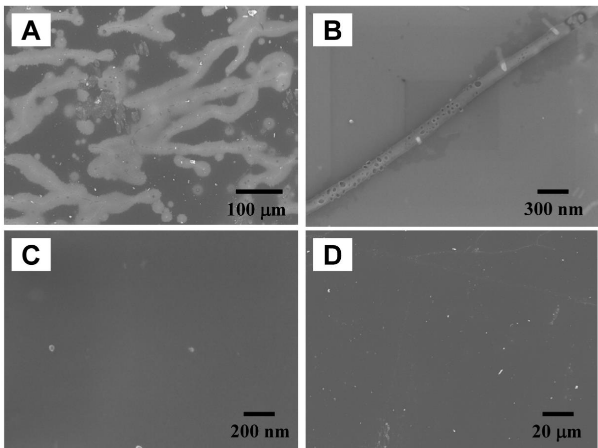
Figura 32 – Micrografias da superfície das membranas PS/SEBS: (a) baixa ampliação (antes do tratamento); (b) elevada ampliação (antes do tratamento); (c) baixa ampliação (depois do tratamento); e (d) PS/SEBS/PAni (depois do tratamento).
