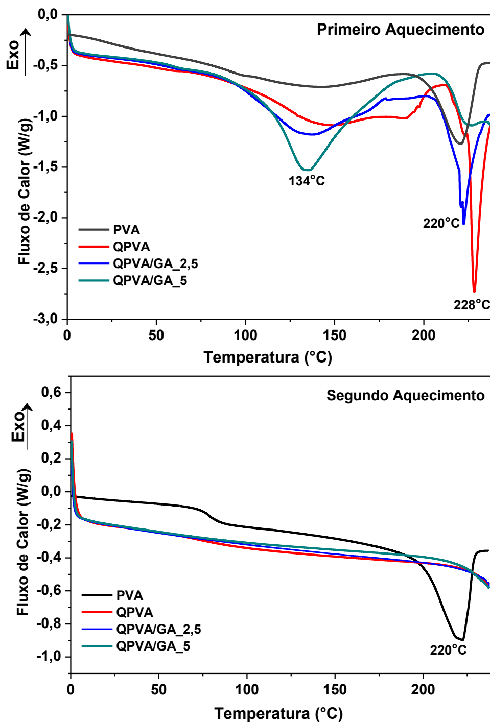
Figura 44 - Termograma DSC das membranas QPVA/GA comparadas com os polímeros individuais no primeiro e segundo aquecimentos.
