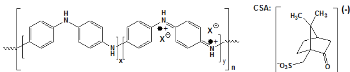
Figura 18 – Estrutura química da PANi dopada com CSA ( \text{X}^- ).
