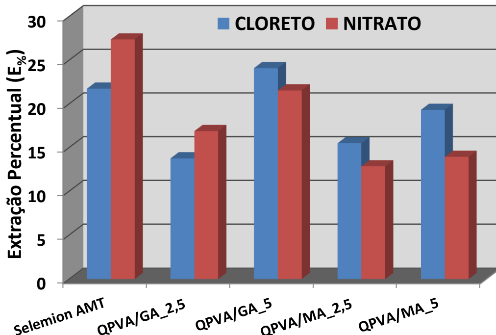
Figura 46 - Extração percentual de cloreto e nitrato para as membranas Selemion ® AMV, QPVA/GA_2,5, QPVA/GA_5, QPVA/MA_2,5 e QPVA/MA_5. Tempo de ensaio 240 min e densidade de corrente 3,5 mA/cm 2 .
