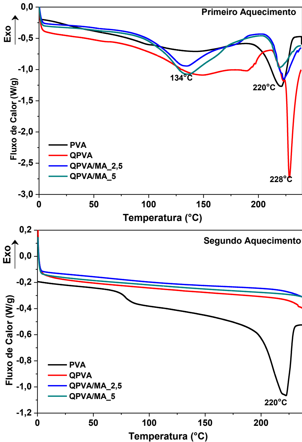
Figura 43 – Termograma DSC das membranas QPVA/MA comparadas com os polímeros individuais no primeiro e segundo aquecimentos.
