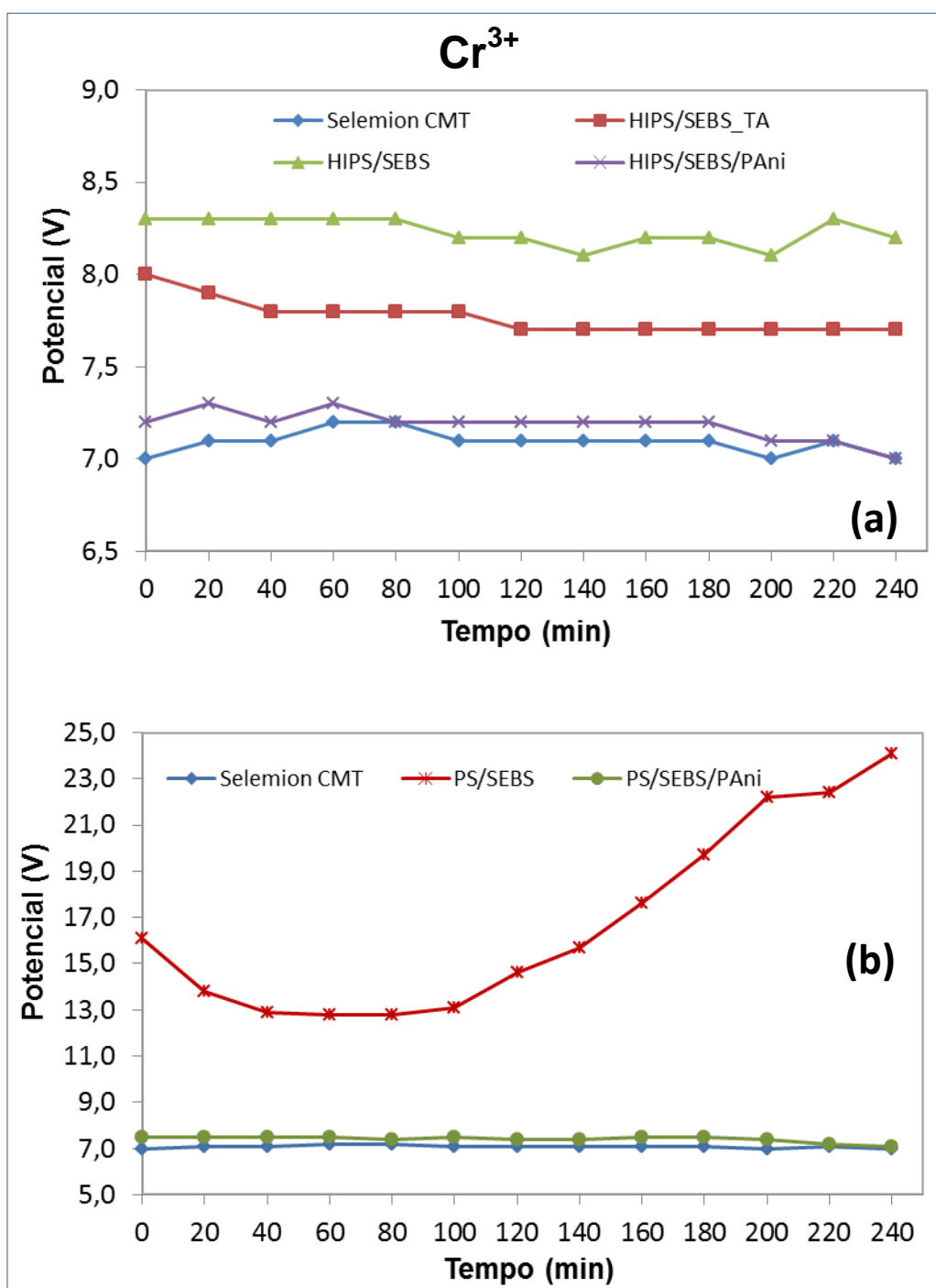
Figura 39 - Potencial elétrico medido durante o ensaio de ED para análise de Cr 3+ : (a) membranas Selemion ® CMT, HIPS/SEBS_TA, HIPS/SEBS e HIPS/SEBS/PAni e (b) membranas Selemion ® CMT, PS/SEBS e PS/SEBS/PAni. Densidade de corrente 3,5 mA/cm 2 .
