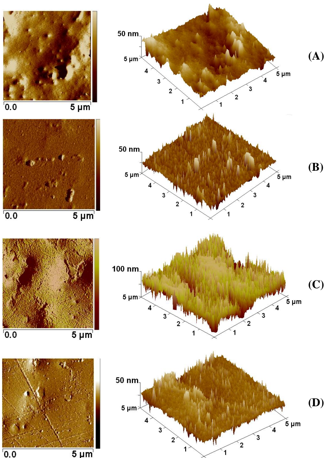
Figura 34 – Imagens topográficas da superfície das membranas: (a) PS/SEBS, (b) PS/SEBS/PAni, (c) HIPS/SEBS e (d) HIPS/SEBS/PAni. Esquerda: Imagem frontal. Direita: Imagem 3D.
