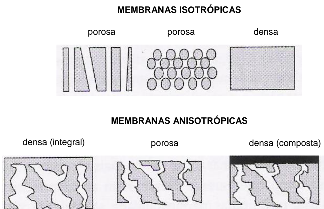
Figura 9 – Representação da seção transversal dos diferentes tipos de morfologia de membranas sintéticas [37].
