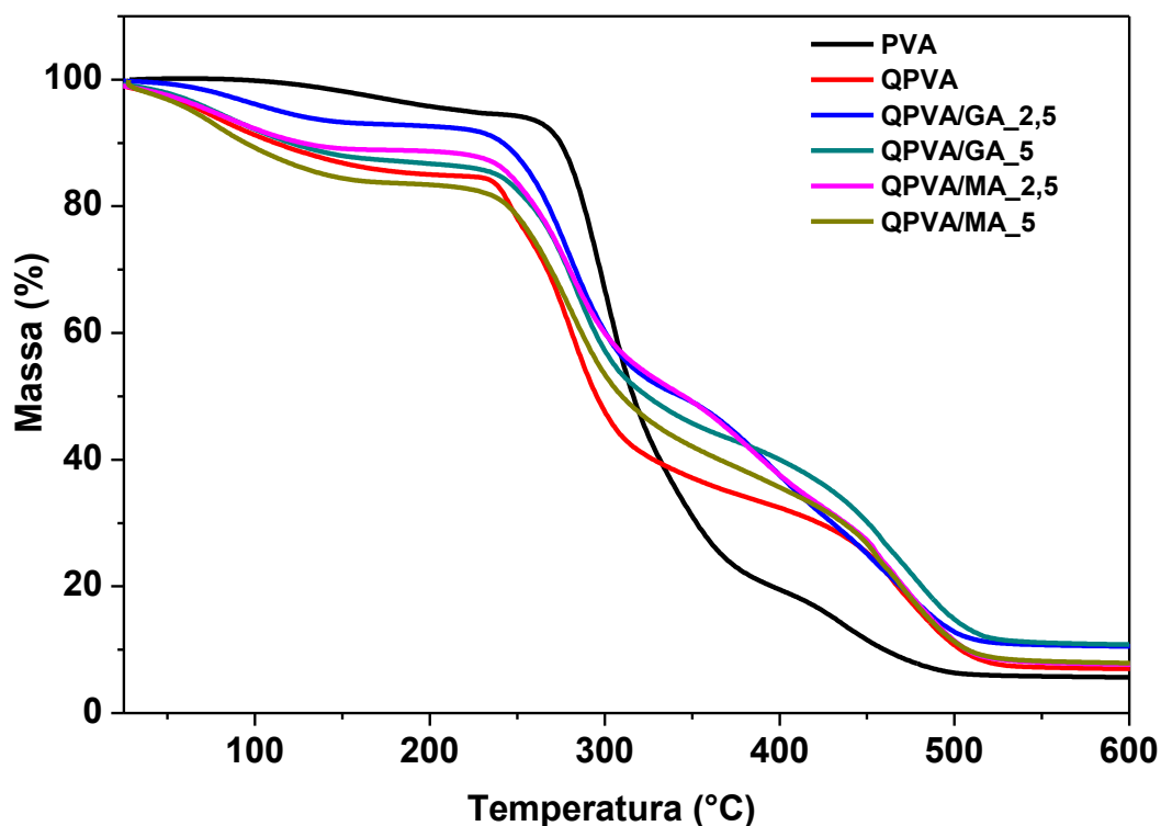
Figura 42 - Análise termogravimétrica das membranas aniônicas produzidas.
