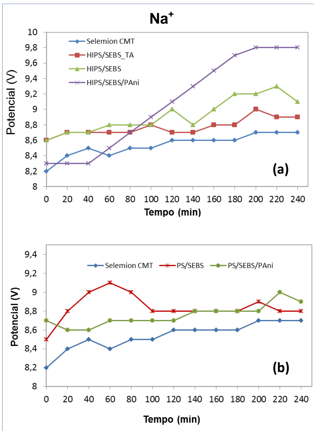
Figura 37 - Potencial elétrico medido durante o ensaio de ED para análise de Na + : (a) membranas Selemion ® CMT, HIPS/SEBS_TA, HIPS/SEBS e HIPS/SEBS/PAni e (b) membranas Selemion ® CMT, PS/SEBS e PS/SEBS/PAni. Densidade de corrente 3,5 mA/cm 2 .
