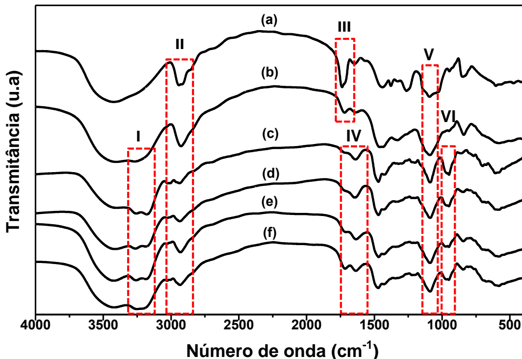
Figura 41 - Espectro FTIR das amostras (a) PVA, (b) QPVA, (c) QPVA/GA_2,5, (d) QPVA/GA_5, (e) QPVA/MA_2,5 e (f) QPVA/MA_5.
