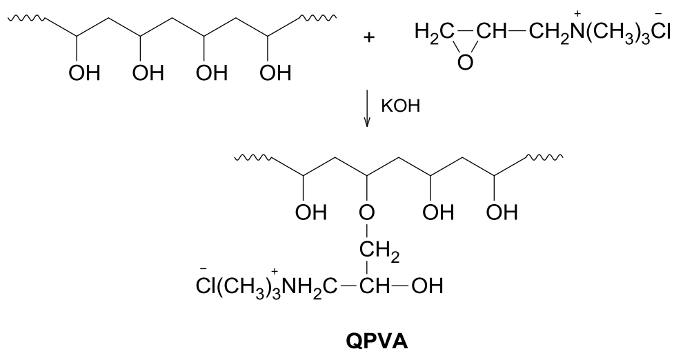
Figura 20 – Sequência da reação para formação do QPVA.
