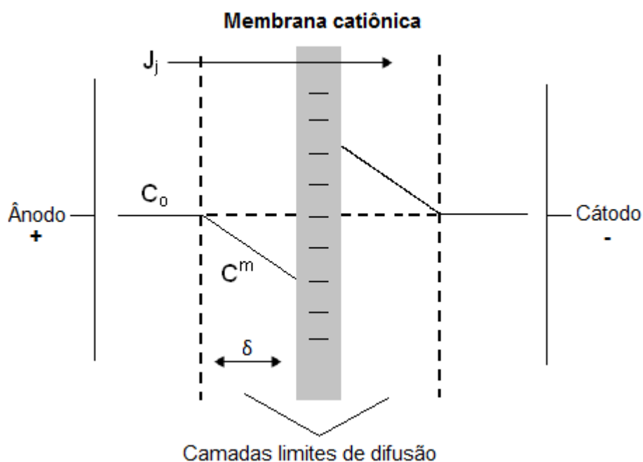
Figura 2 – Perfil da concentração do contra-íon nas camadas de polarização em uma membrana.
