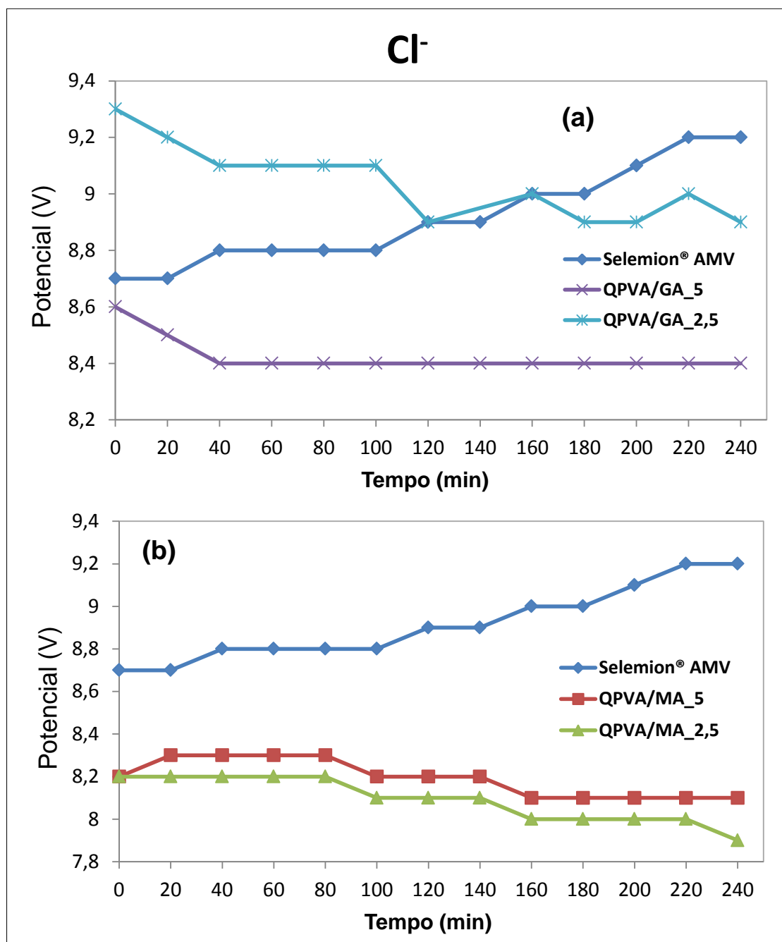
Figura 47 - Potencial elétrico medido durante o ensaio de ED para análise de Cl - : (a) membranas Selemion® AMV, QPVA/GA_5, QPVA/GA_2,5 e (b) membranas Selemion® AMV, QPVA/MA_5, QPVA/MA_2,5. Densidade de corrente 3,5 mA/cm 2 .
