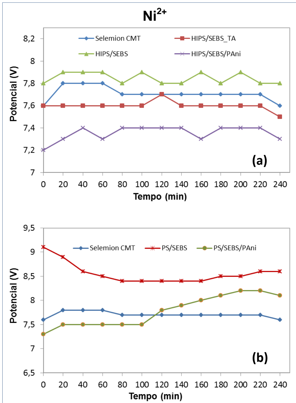
Figura 38 - Potencial elétrico medido durante o ensaio de ED para análise de Ni 2+ : (a) membranas Selemion ® CMT, HIPS/SEBS_TA, HIPS/SEBS e HIPS/SEBS/PAni e (b) membranas Selemion ® CMT, PS/SEBS e PS/SEBS/PAni. Densidade de corrente 3,5 mA/cm 2 .
