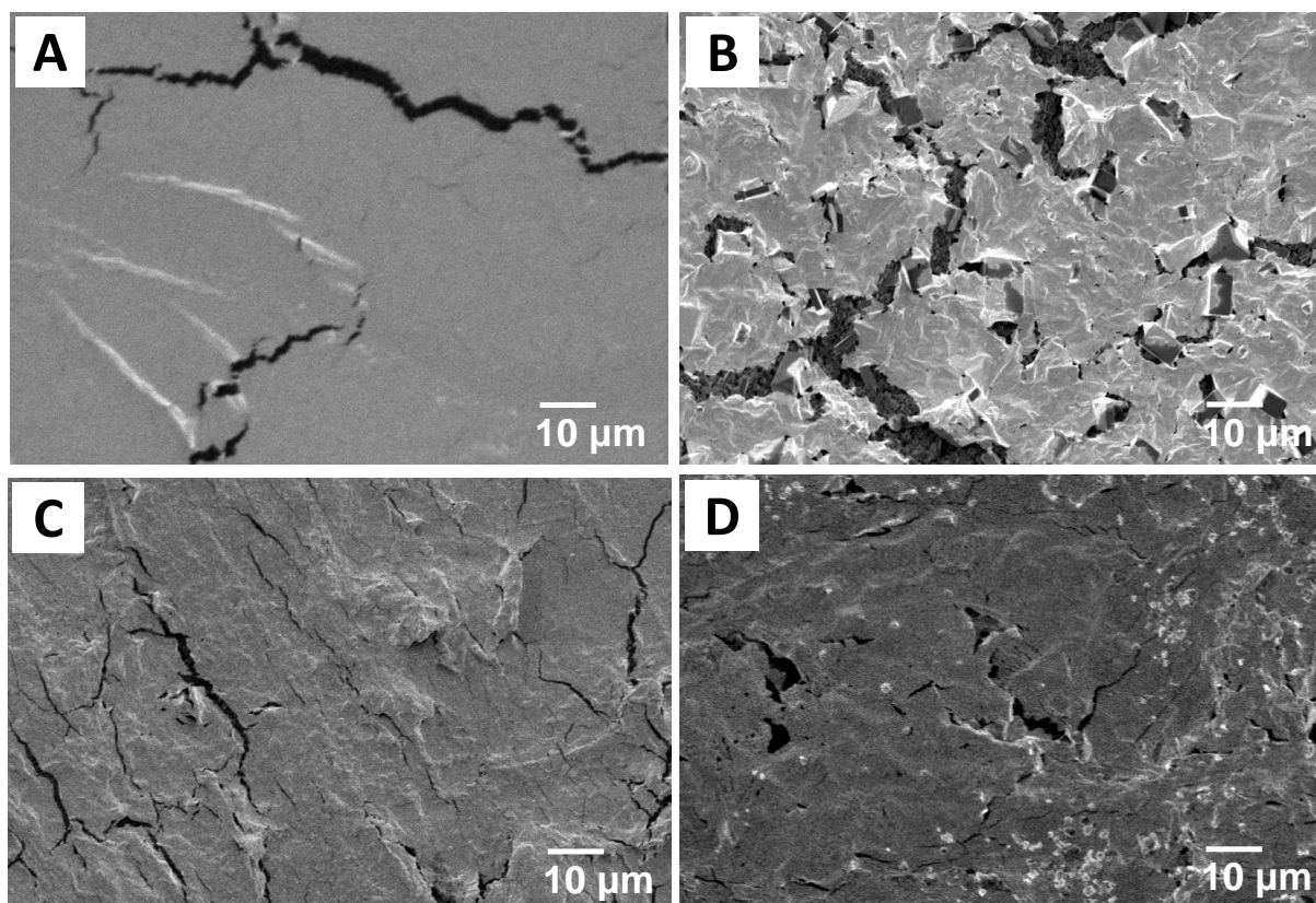
Figura 45 - Micrografia de MEV para as membranas aniônicas: (A) QPVA/GA_2,5 (B) QPVA/GA_5 (C) QPVA/MA_2,5 e (D) QPVA/MA_5. (Magnificação: 10µm)
