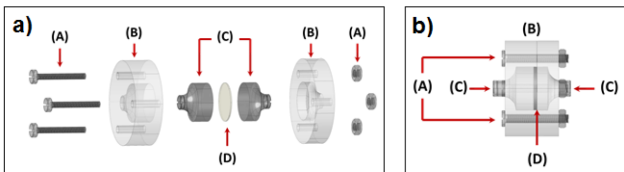
Figura 22 – Sistema usado para medidas de condutividade: (a) Arranjo da célula (A) Parafusos e porcas usados para fixar a célula, (B) Blocos de Teflon®, (C) Eletrodos de contato de aço inoxidável, (D) Membrana polimérica e (b) Célula fechada.
