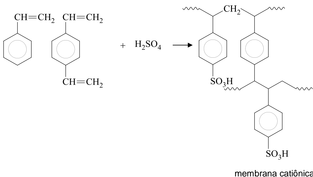
Figura 4 – Esquema de polimerização para obtenção de uma membrana catiônica [40].
