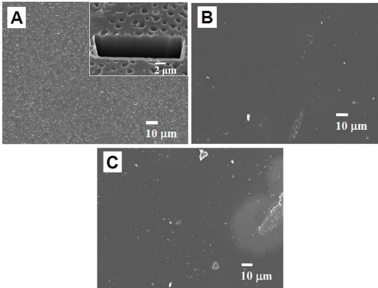
Figura 31 – Micrografia de MEV para os polímeros individuais usados como referência: (a) PS, (b) HIPS e (c) SEBS. A inserção em uma parte de alta ampliação denota uma imagem mostrando a porosidade dentro do filme de PS preparado por evaporação do solvente e seco a temperatura ambiente (escala: 2 \mu\text{m} ).
