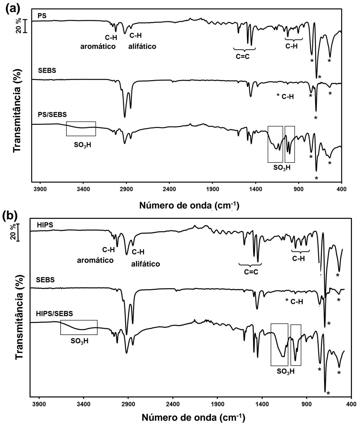
Figura 27 – Espectros FTIR-ATR (a) polímeros individuais de PS e SEBS e da membrana sulfonada de PS/SEBS; (b) polímeros individuais de HIPS e SEBS e da membrana sulfonada de HIPS/SEBS. Asterisco indica os estiramentos das vibrações de C-H “no e fora” do plano.
