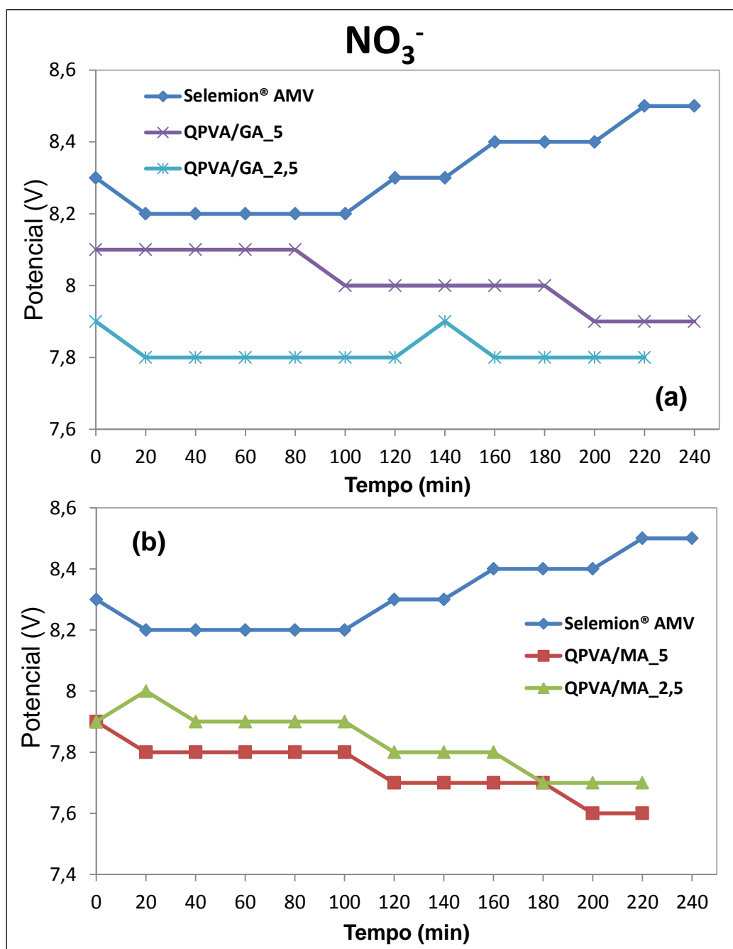
Figura 48 - Potencial elétrico medido durante o ensaio de ED para análise de NO 3 - : (a) membranas Selemion® AMV, QPVA/GA_5, QPVA/GA_2,5 e (b) membranas Selemion® AMV, QPVA/MA_5, QPVA/MA_2,5. Densidade de corrente 3,5 mA/cm 2 .
