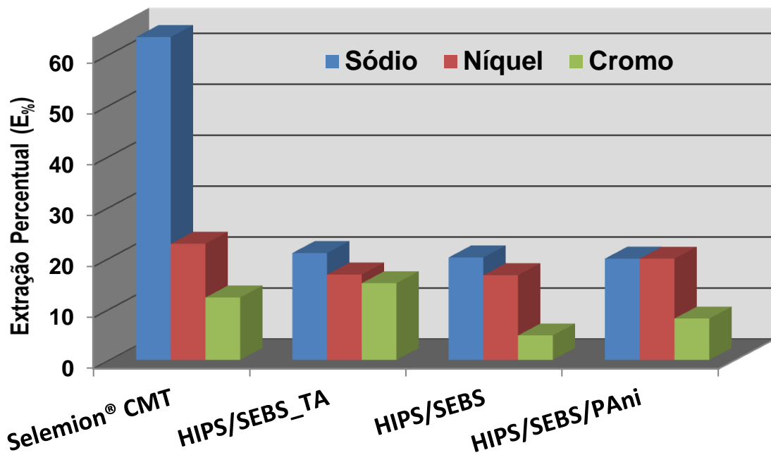
Figura 36 - Extração percentual de sódio, níquel e cromo para as membranas Selemion® CMT, HIPS/SEBS_TA, HIPS/SEBS e HIPS/SEBS/PAni. Tempo de ensaio 240 min e densidade de corrente 3,5 mA/cm 2 .
