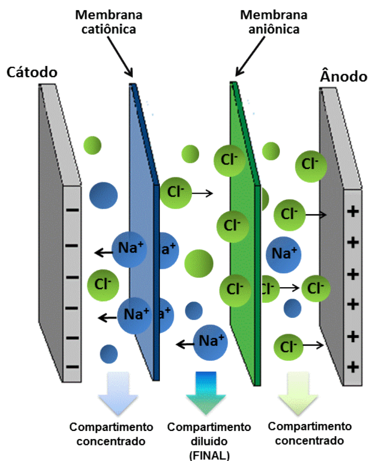
Figura 1 – Representação esquemática de um sistema de eletrodialise, contemplando um par de membranas (catiônica e aniônica).
