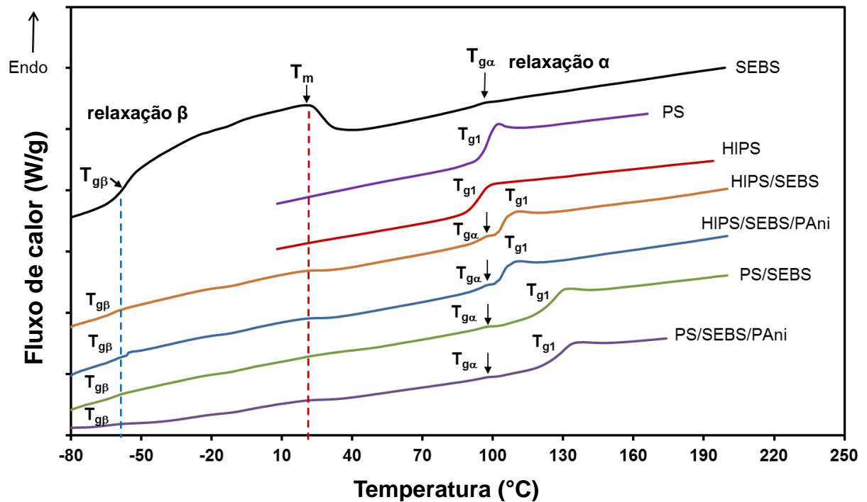
Figura 28 – Termogramas de DSC das membranas PS/SEBS e HIPS/SEBS, comparadas com os polímeros individuais (PS, SEBS e HIPS). Todas as curvas se referem ao segundo aquecimento.
