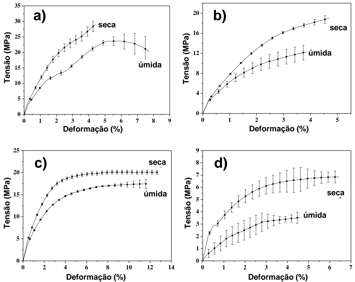
Figura 30 – Curvas de tensão x deformação para as membranas previamente secas em estufa a vácuo com temperatura de 60°C (seca) e expostas a câmara úmida (TU 100%, úmida): a) PS/SEBS, b) PS/SEBS/PAni, c) HIPS/SEBS e d) HIPS/SEBS/PAni.
