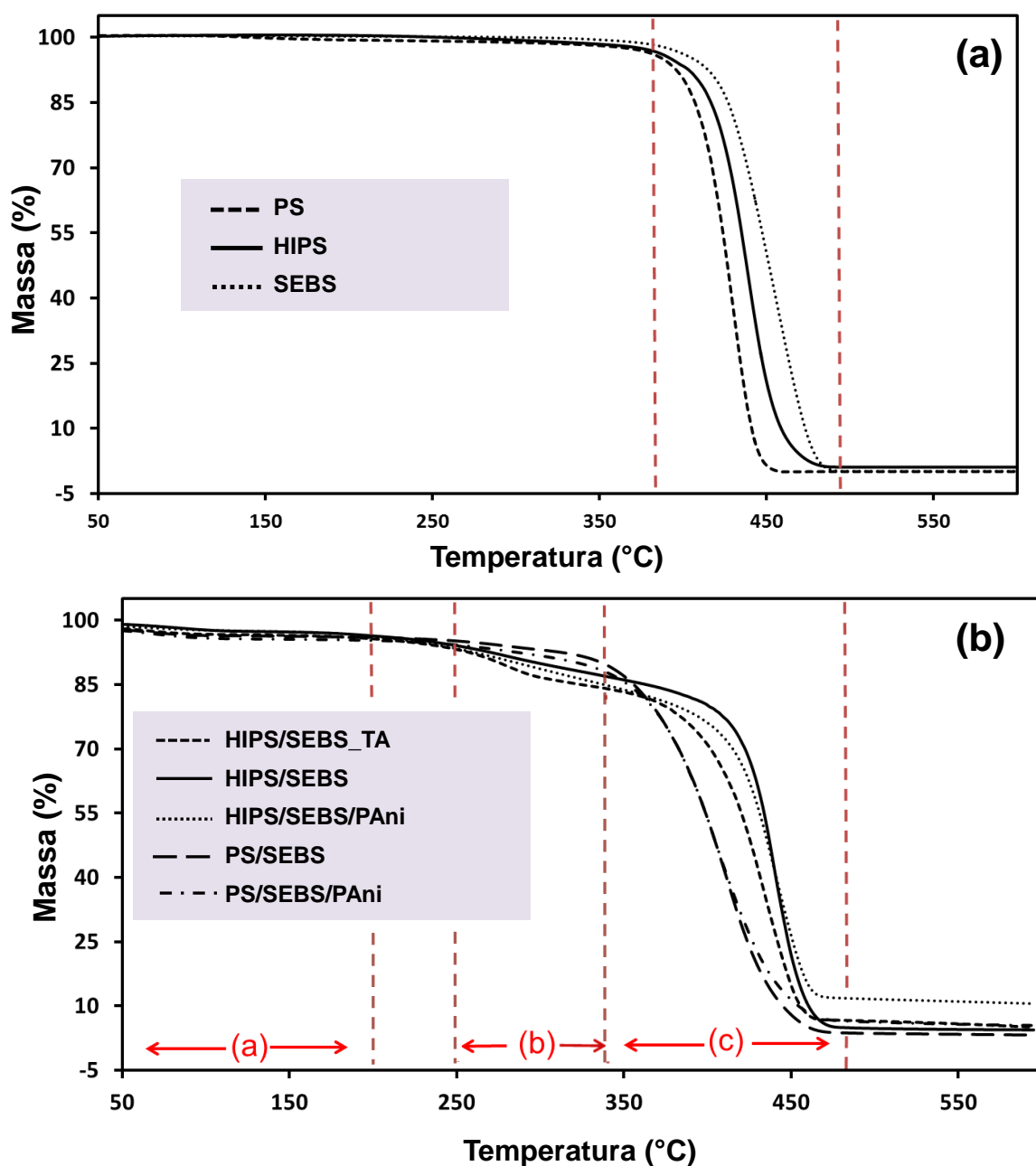
Figura 29 – Análise termogravimétrica das (a) amostras individuais dos polímeros PS, HIPS e SEBS e (b) membranas HIPS/SEBS_TA, HIPS/SEBS, HIPS/SEBS/PAni, PS/SEBS e PS/SEBS/PAni.
