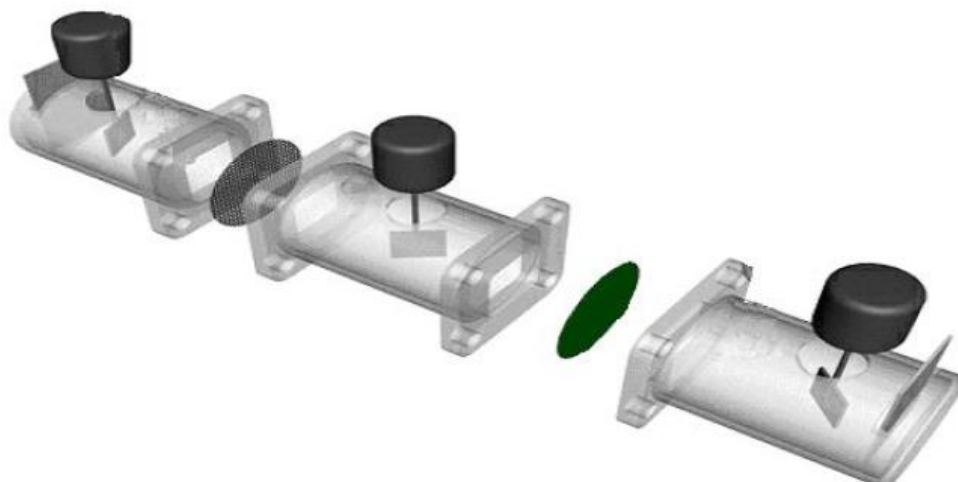
Figura 24– Célula de três compartimentos usada para eletrodialise.
