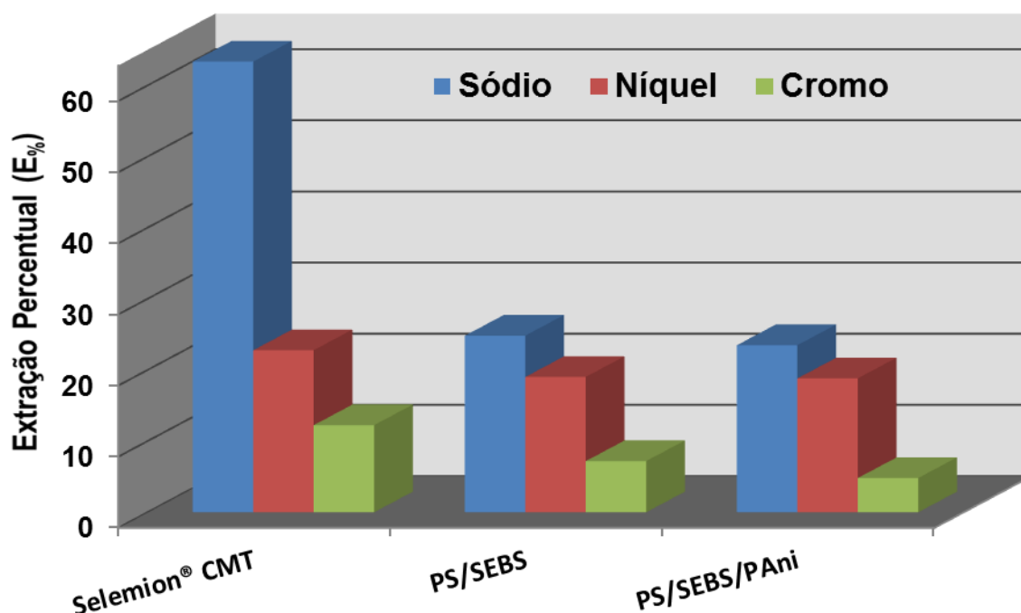
Figura 35 - Extração percentual de sódio, níquel e cromo para as membranas Selemion® CMT, PS/SEBS e PS/SEBS/PAni. Tempo de ensaio 240 min e densidade de corrente 3,5 mA/cm 2 .
