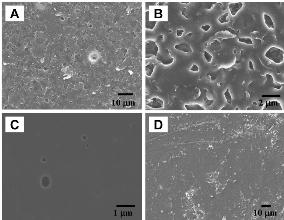
Figura 33 – Micrografias das membranas HIPS/SEBS: (a) baixa ampliação (antes do tratamento), (b) elevada ampliação (antes do tratamento), (c) baixa ampliação (depois do tratamento) e (d) HIPS/SEBS/PAni (depois do tratamento).
