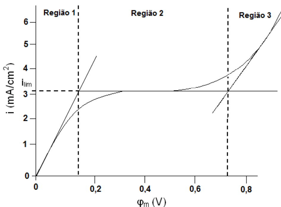
Figura 3 - Curva corrente-potencial para uma membrana íon seletiva [29].
