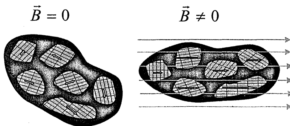
Figura II.1.1. Alineament de partícules isotròpies de Nd-Fe-B sota un camp magnètic.
