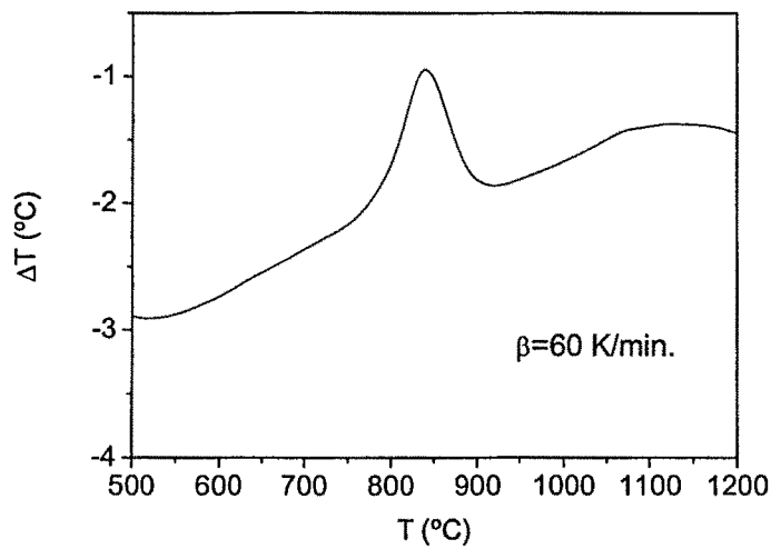
Figura II.3.12. Corba ATD de nanopartícules d' \epsilon - \text{Fe}_2\text{O}_3 en atmosfera d'aire.
