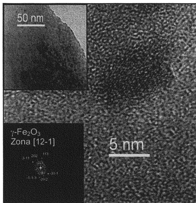
Figura II.3.3. Imatges al MET del xerogel recuït fins a 700 °C. La transformada de Fourier de la imatge d'alta resolució indica que les nanopartícules són de \gamma - \text{Fe}_2\text{O}_3 .
