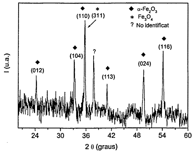
Figura II.3.13. Espectre de DRX de la pols obtinguda després de l'experiment d'ATD en què nanopartícules d' \epsilon - \text{Fe}_2\text{O}_3 es van escalfar fins a 1200 °C en atmosfera d'aire.
