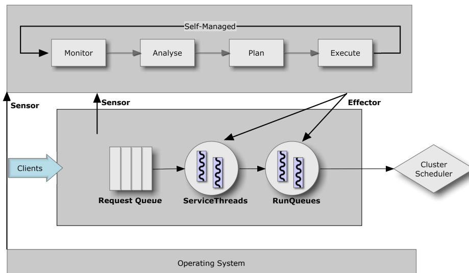
Figura 3.16: Diagrama del prototipo autónomo.
