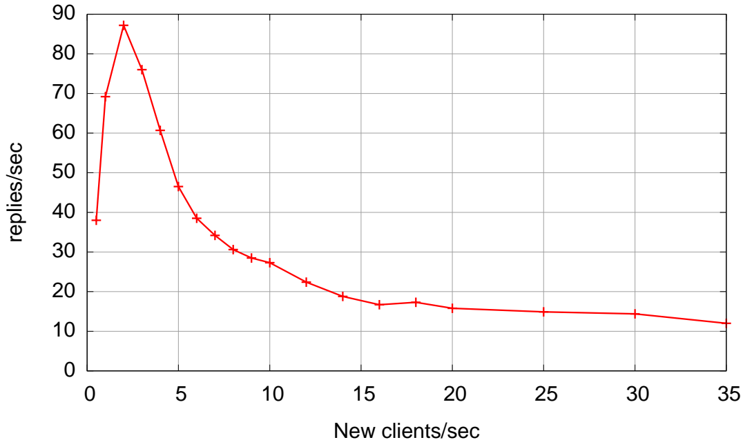
Figura 2.1: Rendimiento del servidor de aplicaciones Tomcat sobrecargado.
