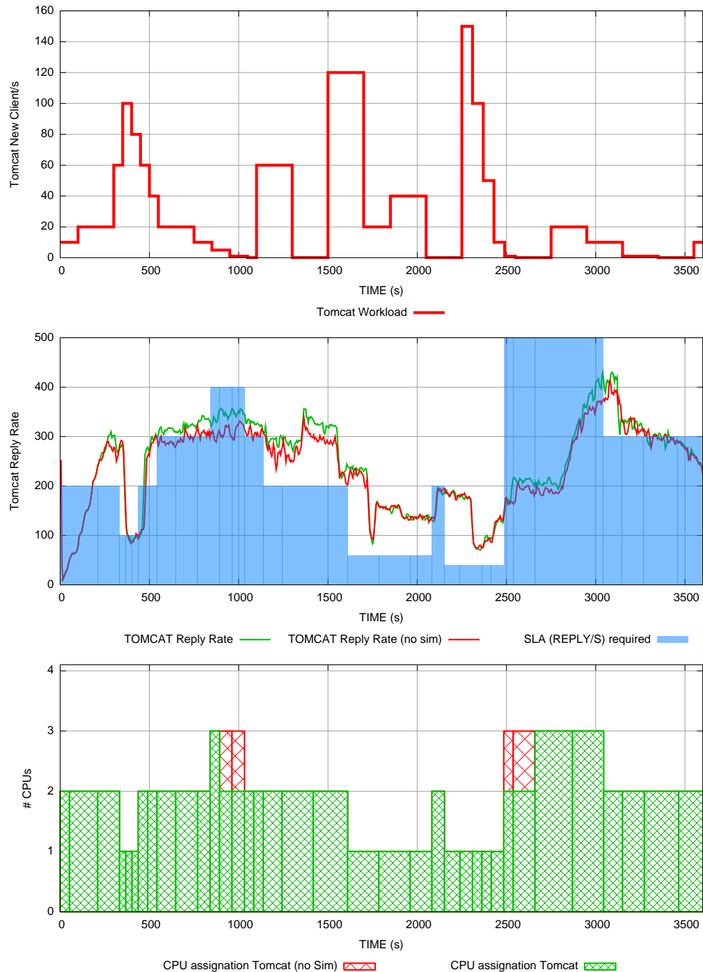
Figura 6.7: Ejecución de un entorno heterogéneo con un gestor de recursos sin predicción (se utiliza una política estática). Nótese la diferencia de asignación de procesadores sin producir beneficios en el throughput.
