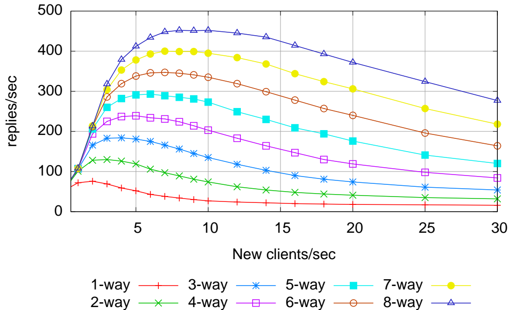
Figura 2.7: Throughput predcido de Tomcat en un multiprocesador.
