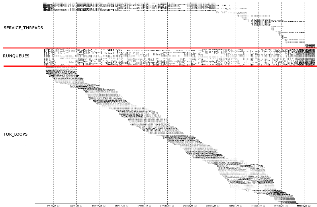
Figura 3.6: Traza Paraver que muestra el comportamiento del sistema cuando estamos enviando trabajos que sobrecargan la CPU.
