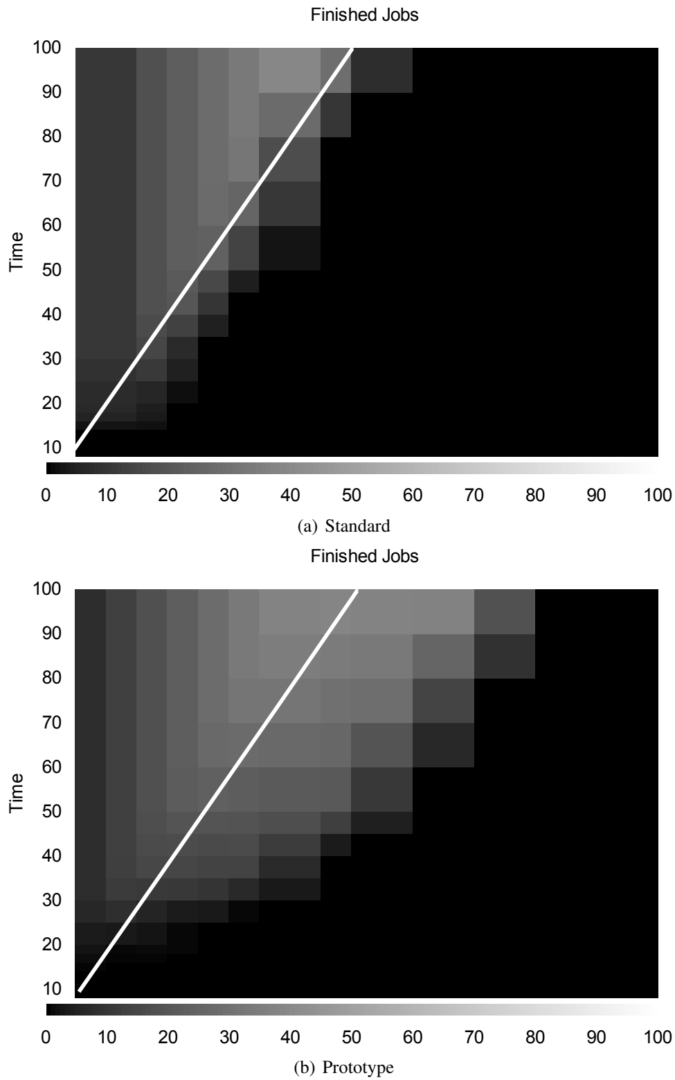
Figura 3.20: Trabajos finalizados usando 1 procesador en el middleware original y nuestro prototipo. Con una línea blanca frontera teórica para la ejecución de todos los trabajos.
