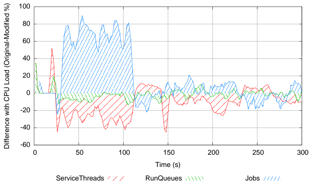
Figura 3.15: Diferencia del consumo de CPU entre las dos propuestas (original-modificado).
