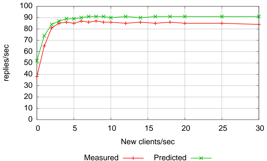
Figura 2.6: Throughput de Tomcat con control de admisión, comparación entre el sistema experimental y el modelo predicho (1 CPU).
