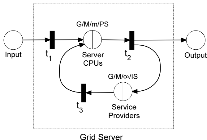
Figura 5.3: Modelo QPN de un servidor Grid .
