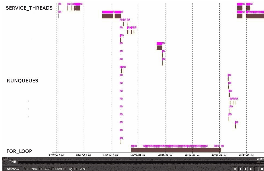
Figura 3.7: Traza con el comportamiento de la ejecución de 1 trabajo; los cambios de contexto están marcados con una bandera.
