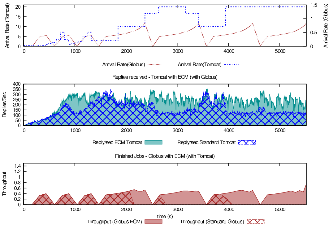
Figura 4.3: De arriba a abajo: Carga de Tomcat y de Globus, respuestas por segundo de un Tomcat sin autogestión a otro con ECM y throughput de Globus estandar comparado con el throughput obtenido con ECM. Las dos aplicaciones están ejecutándose a la vez usando ECM.
