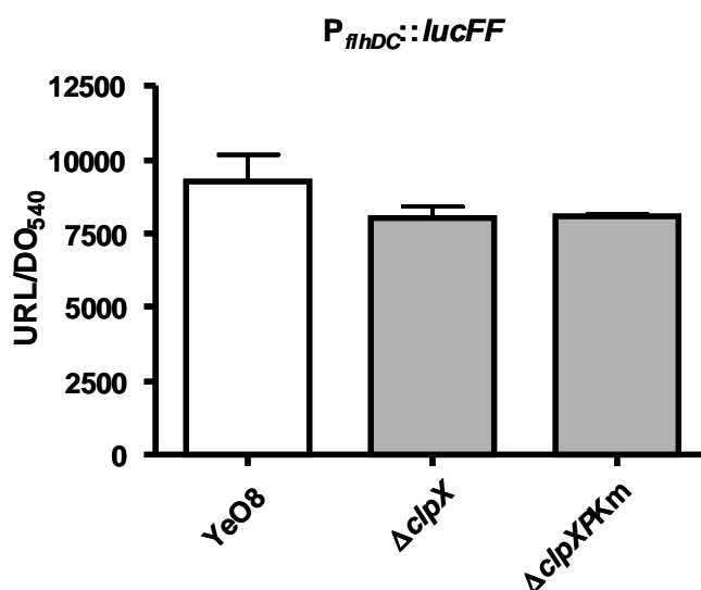
Figura 22. Análisis de la transcripción de flhDC en los mutantes YeO8- \Delta clpX y YeO8- \Delta clpXP. Expresión de flhDC en YeO8, YeO8- \Delta clpX ( \Delta clpX) y YeO8- \Delta clpXPkm ( \Delta clpXPkm). Los resultados corresponden a tres experimentos independientes realizados por quintuplicado.
