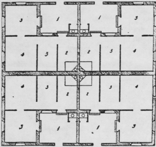
Fig. 78.—Grupo de cuatro casas para obreros agrícolas.—Plano general.—1, patio; 2, cocinas; 3, 4 y 5, dormitorios.
