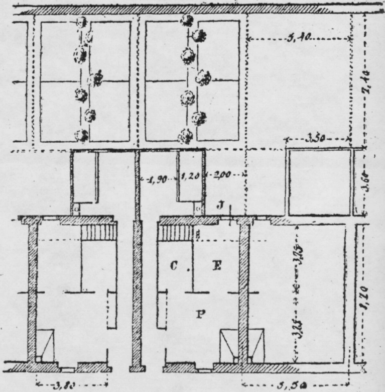
Planta baja
