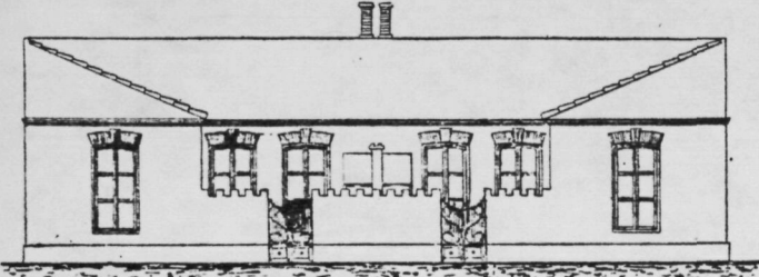
Fig. 76.—Grupo de cuatro casas para obreros agrícolas, del autor de este libro.—Fachada principal.
