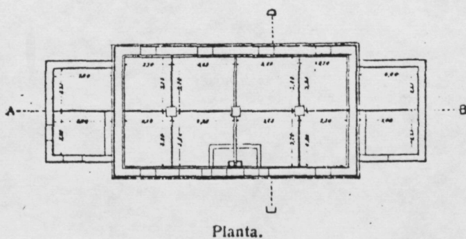
Planta.
