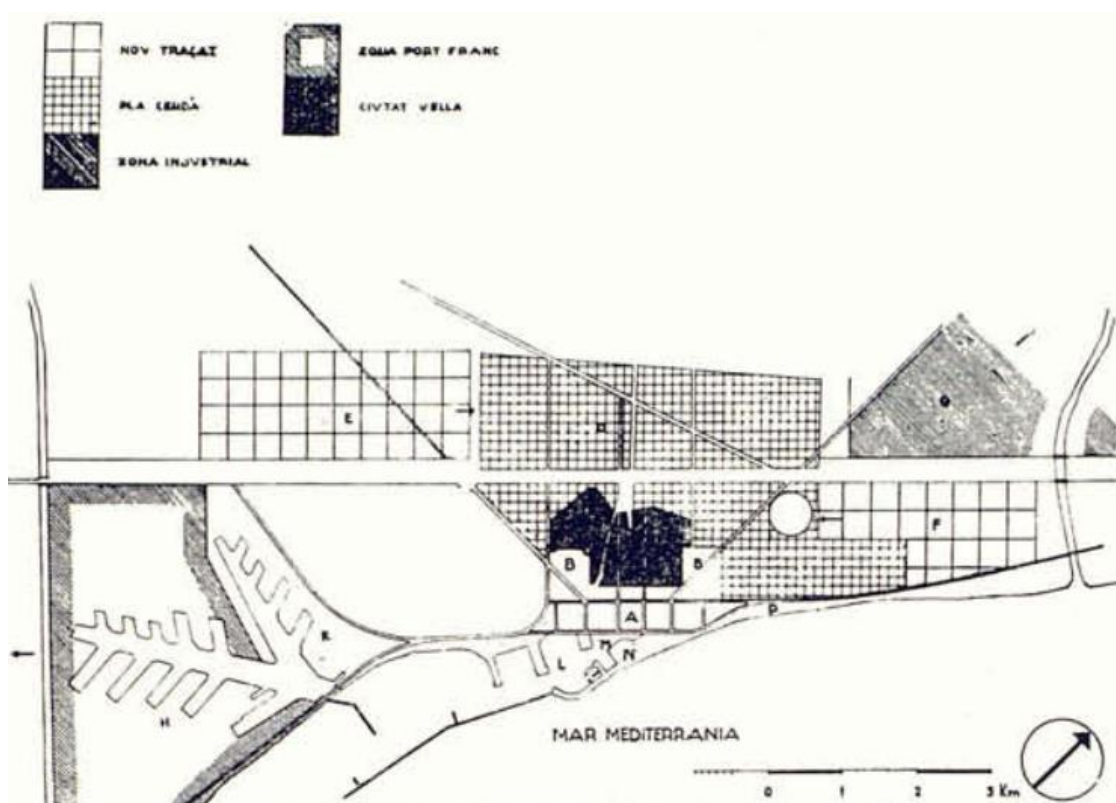
Mapa de la zonificació proposada pel GATCPAC (Juliol de 1934).
