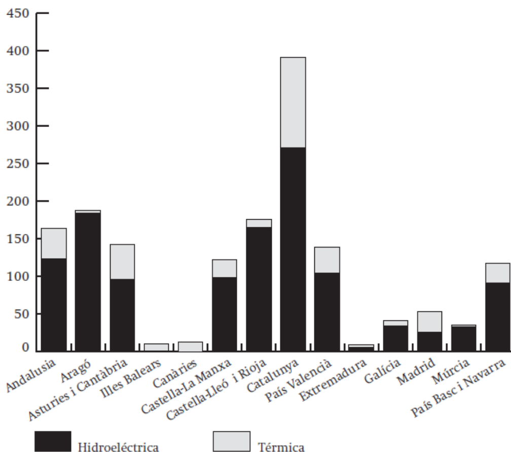
Potència instal·lada per regions, 1935 (Mw)
