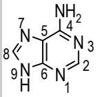
Adenina, Ade
