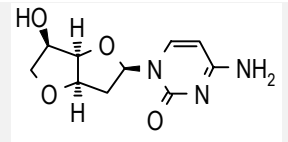
Citosina, Cyt
