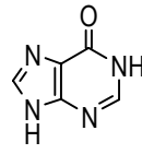
Hypoxantina, Hyp
