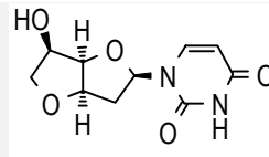
Uracil, Ura
