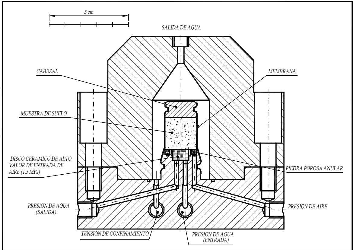
Figura 3.18 Esquema básico de la Mini-célula isotrópica rígida con control de succión.
