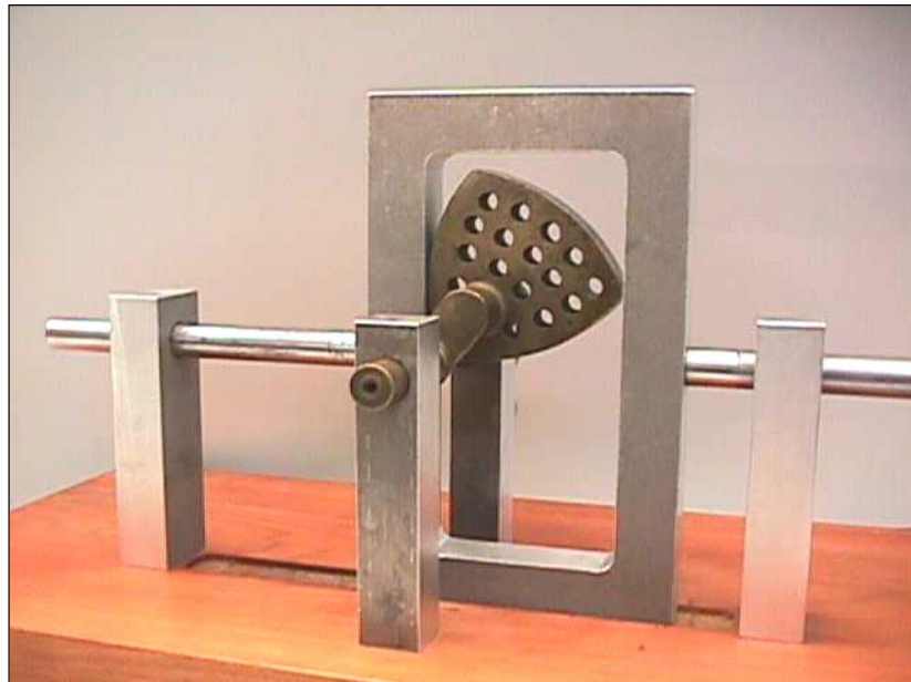
Fig. A-2. Maqueta de leva de anchura constante con doble palpador plano translatorio
