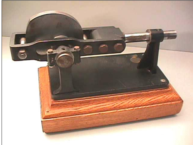
Fig. A-3. Maqueta de leva de anchura constante con doble palpador de rodillo transitorio
