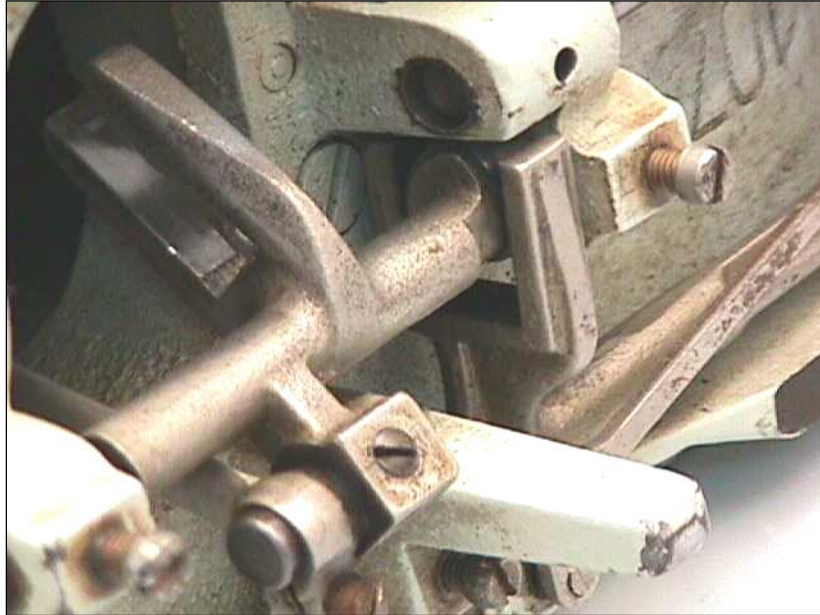
Fig. A-5. Leva de anchura constante con palpador rotatorio utilizada en máquinas de coser
