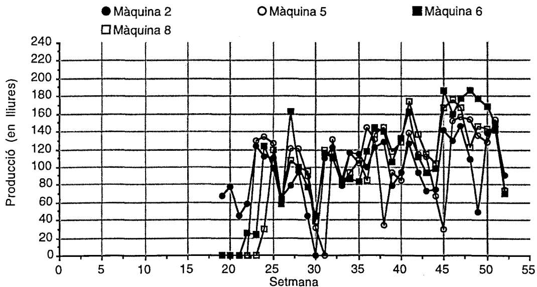
GRÀFIC 6.6.: FÀBRICA DE FILATS DE COTÓ DE FERRER GERMANS A LA MASÓ (ALT CAMP): PRODUCCIÓ SETMANAL DE FIL DE "FUSADAS" DE LES MÀQUINES/FILADORES 2, 5, 6 i 8 (05-05-1850/29-12-1850)
