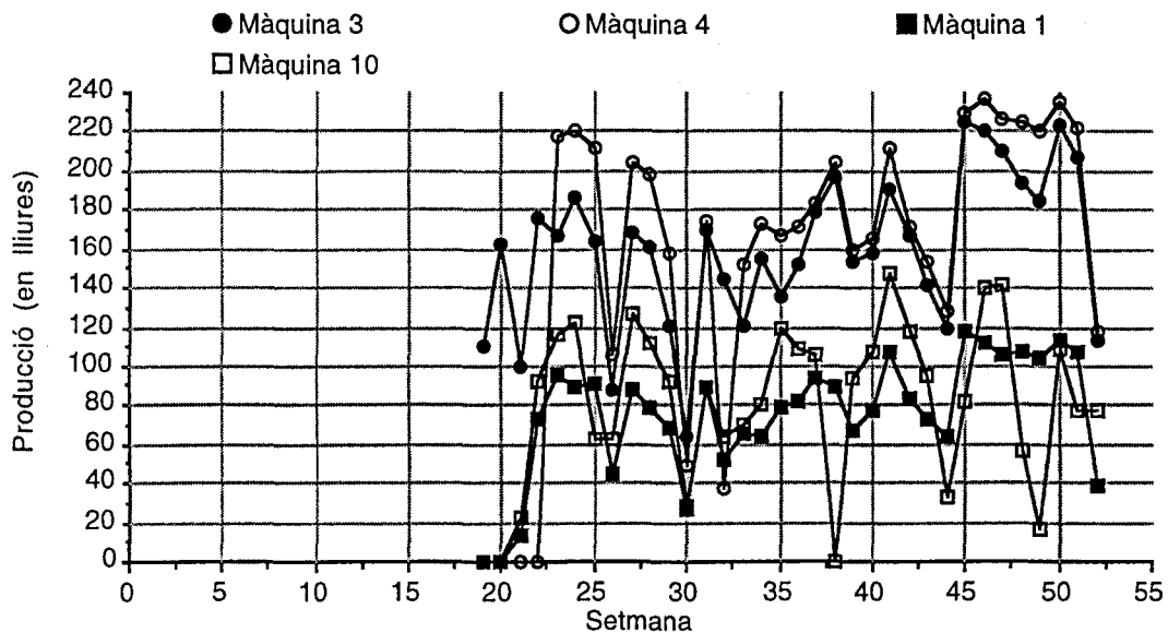
GRÀFIC 6.5.: FÀBRICA DE FILATS DE COTÓ DE FERRER GERMANS A LA MASÓ (ALT CAMP): PRODUCCIÓ SETMANAL DE FIL DE "FUSADAS" DE LES MÀQUINES/FILADORES 1, 3, 4 i 10 (05-05-1850/29-12-1850)
